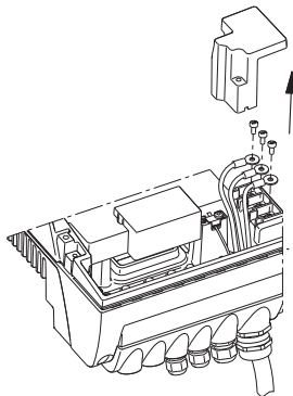
31-сурет Күш сымдарын өшіру
