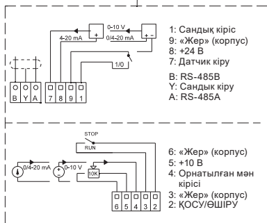
7-сурет TPED 2000 сериялы сорғыларының клеммалары
