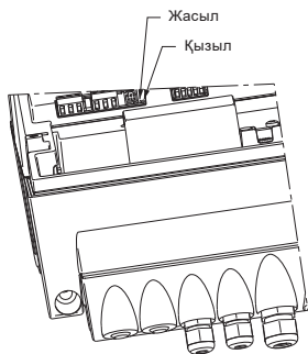
30-сурет Үш фазалы электр қозғалтқыштардан тұратын сорғылардағы жарық индикаторлары. Сонымен қатар, сорғыда кірістірілген реле арқылы потенциалсыз сигнал шығысы бар.
