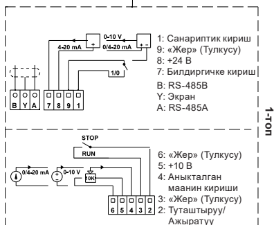
6-сүр. TPE 2000 сериясындагы соргучтардын клеммалары
