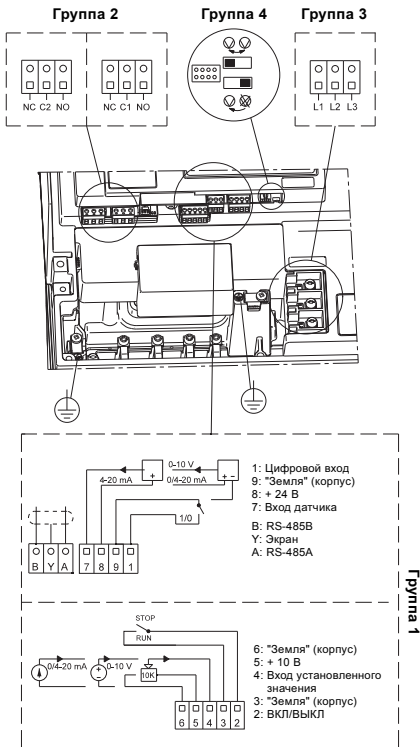
Рис. 7 Клеммы насосов TRPED серии 2000
