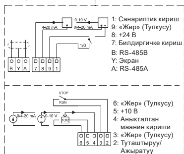
7-сүр. TPED 2000 сериясындагы соргучтардын клеммалары
