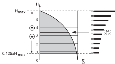
Рис. 20 Насос в режиме регулирования с постоянным напором
