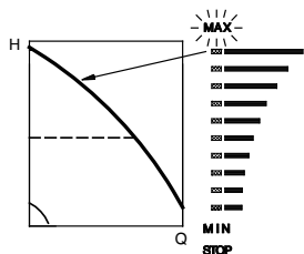
Рис. 21 Макс. характеристика
