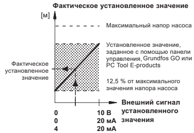
Рис. 28 Зависимость между фактическим установленным значением и внешним сигналом установленного значения при регулировании с постоянным напором
