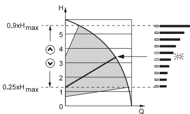
19-сурет Пропорционалды реттелмелі ағынды сорғы
