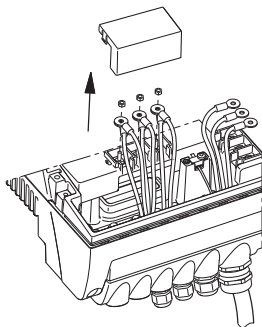
32-сурет Қозғалтқыштың қуат сымдарын өшіру
