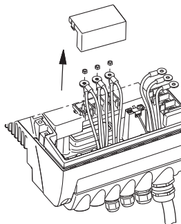
Рис. 32 Отключение проводов питания двигателя
