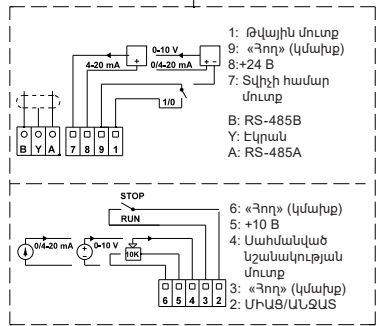
Նկար 6 2000 սերիայի TPE պոմպի սեղմակներ
