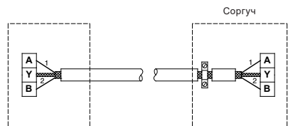
10-сүр. 2 тарамыштуу экрандаштырылган кабели туташтыруу
