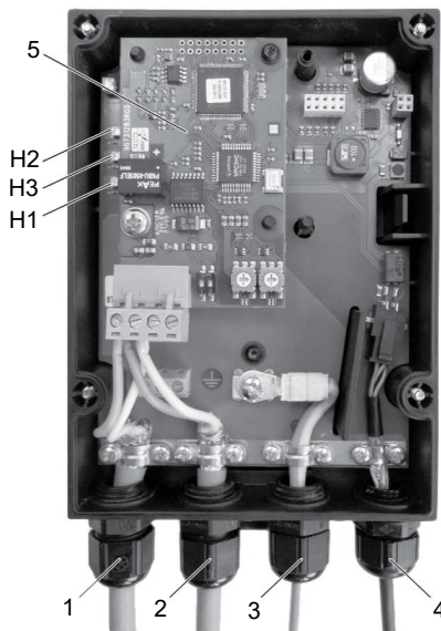
Состав модуля E-vox
