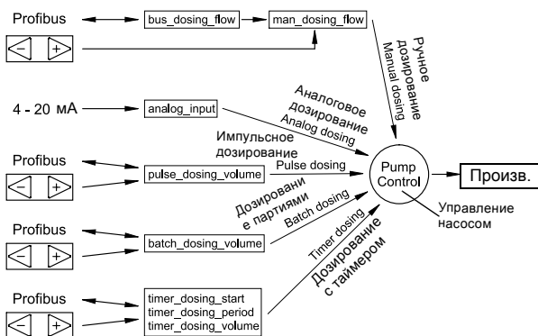
Рис. 4 Пять режимов управления и элементы данных, используемые для генерирования фактической производительности
